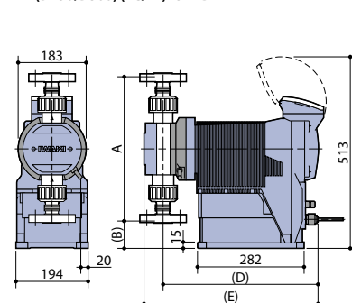
IX- (D150/D300) S6R - RF
